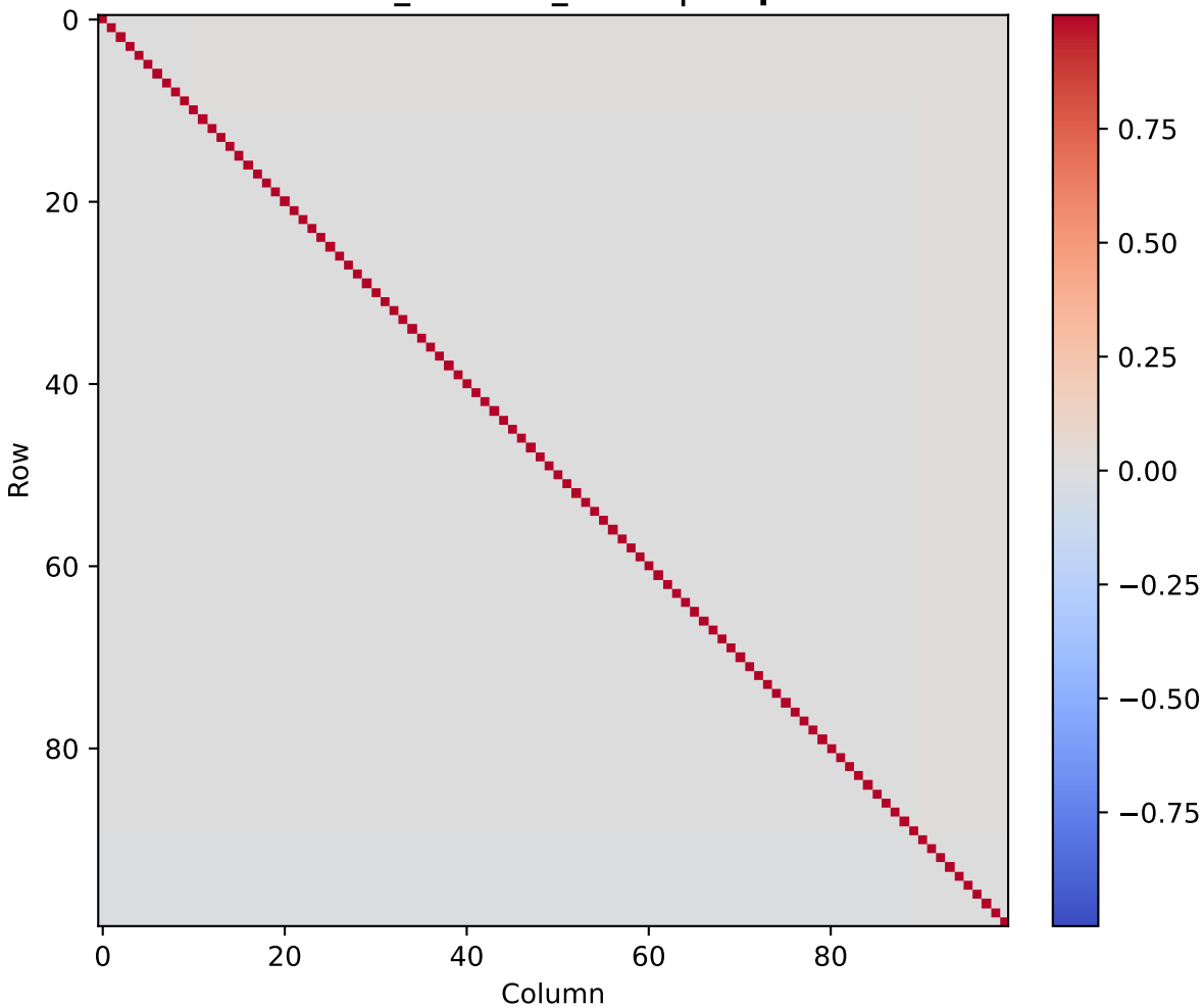
muon_random_small | step 3
